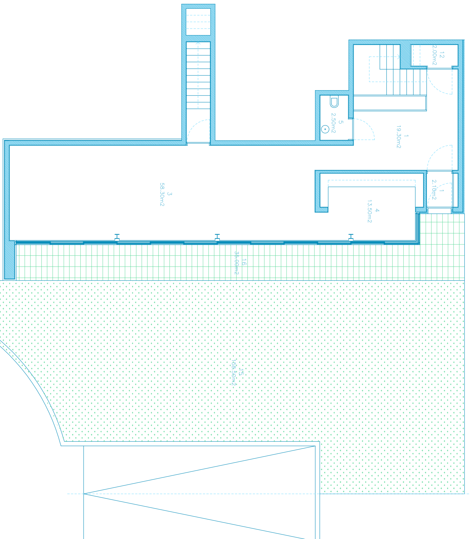
PLANTA PISO -1
